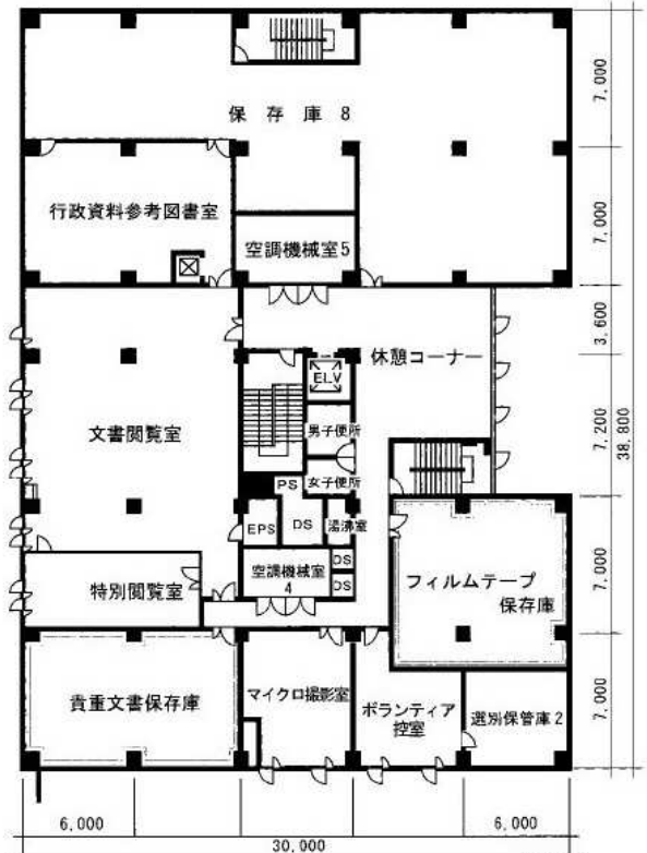
2階平面図
