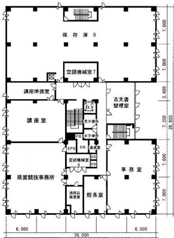
3階平面図
