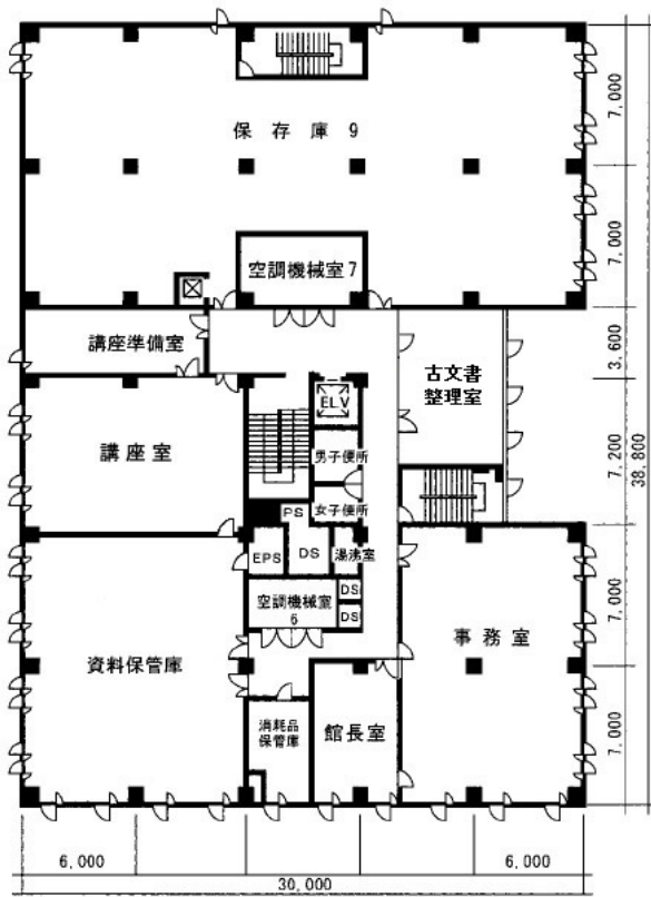
3階平面図
