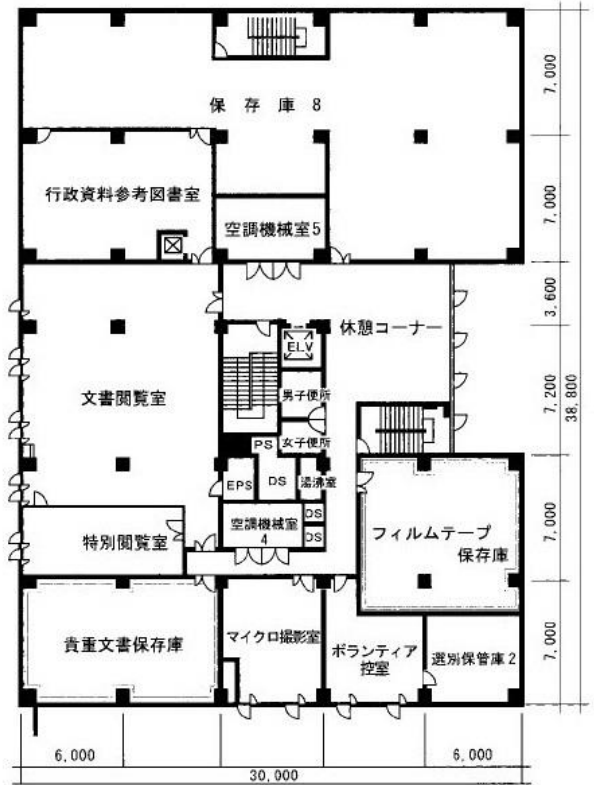
2階平面図
