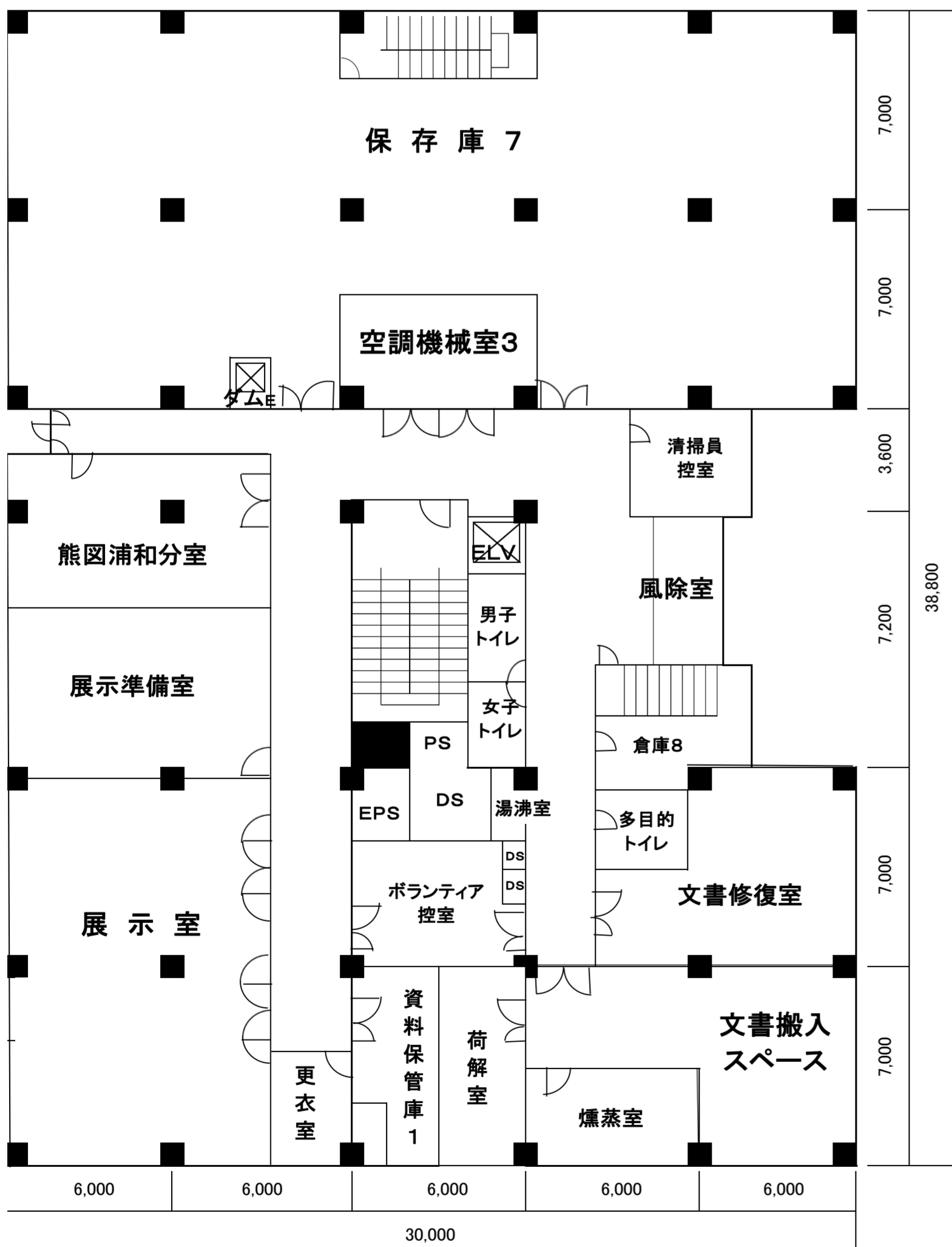
1階平面図
