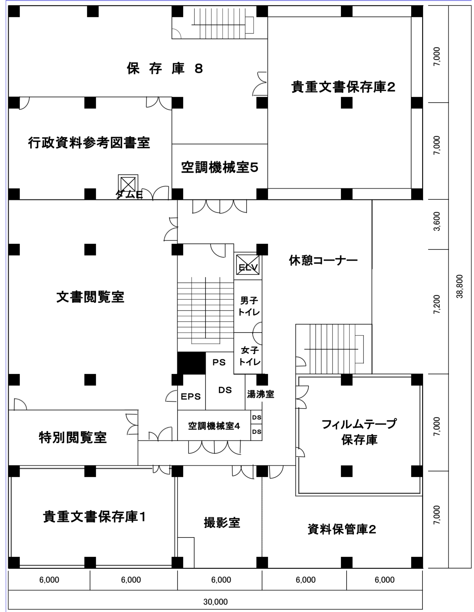
2階平面図
