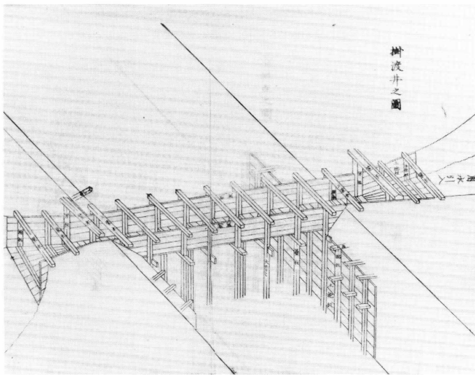
▲ 18 堤防・橋組立之図一掛渡井一
