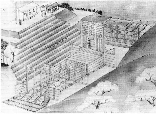
◀ 21 明治年間元塚樋管伏替図(部分)
