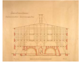
日本练瓦深谷上敷免工厂霍夫曼窑的截面图（日本练瓦制造株式会社文书 136 埼玉县指定文化财产）
